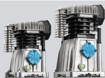
Cabezales ABAC A29(B)-A39(B) con superiores características
